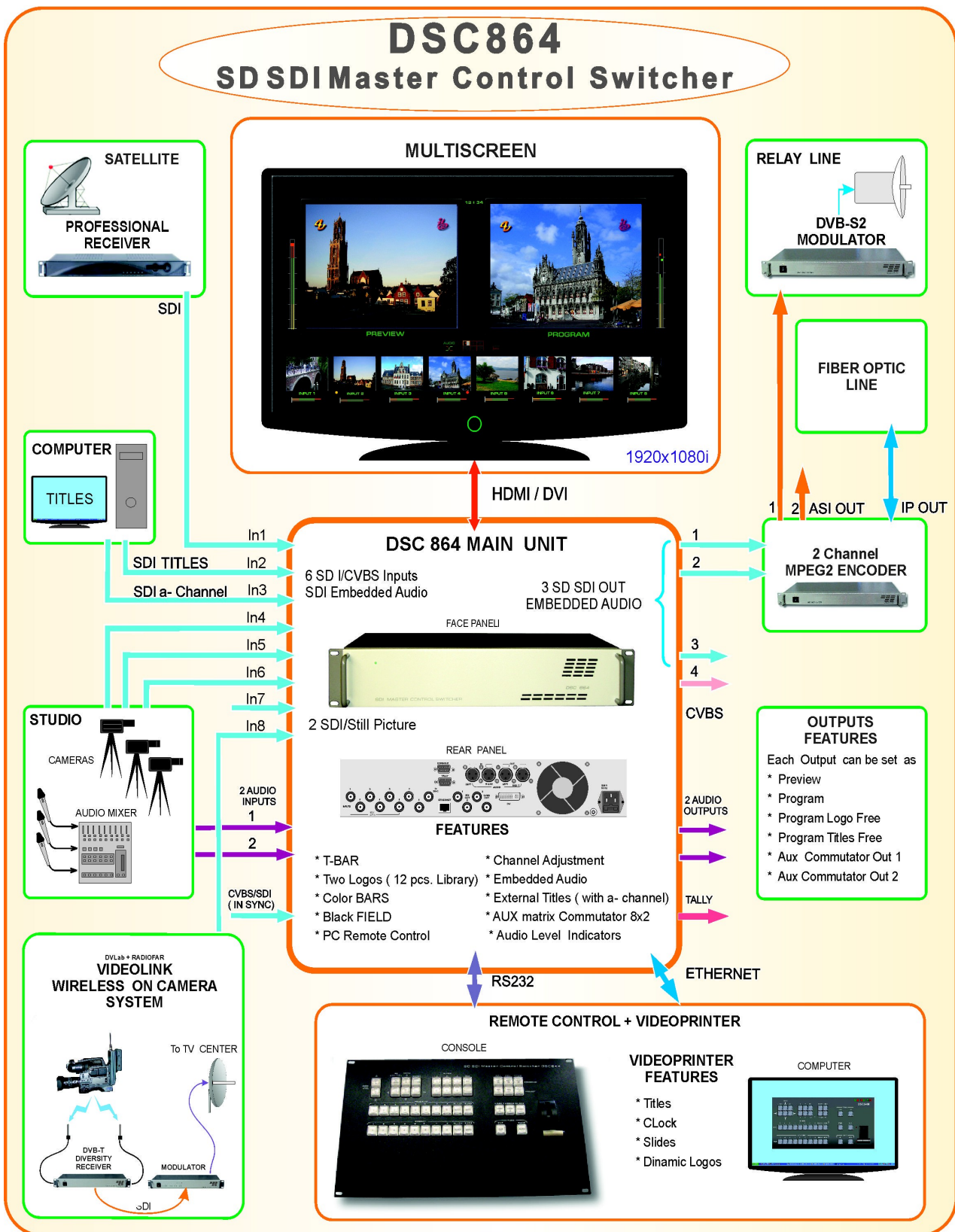
Cxema 2.
